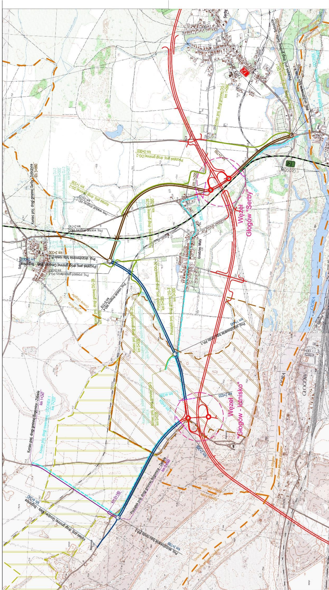
Koncepcja przebiegu dróg do parku przemysłowego
