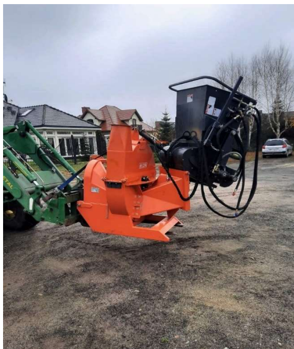
Rębak do gałęzi
