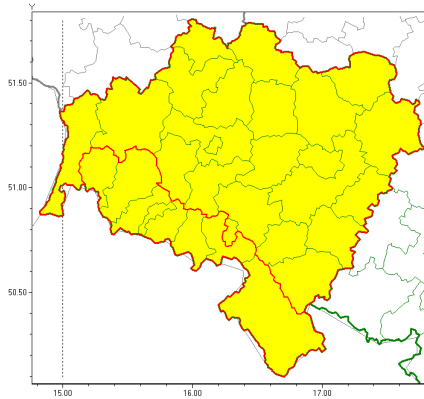
Silny wiatr 2022-02-01 11:25
