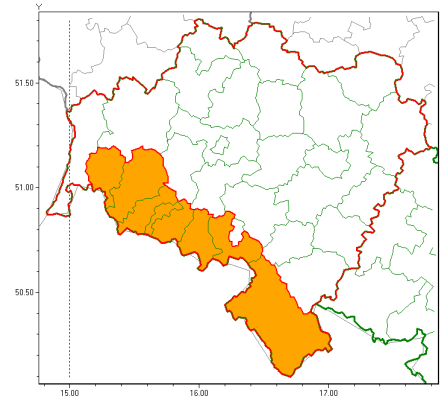
Zawieje/zamiecie śnieżne 2022-02-01 11:25
